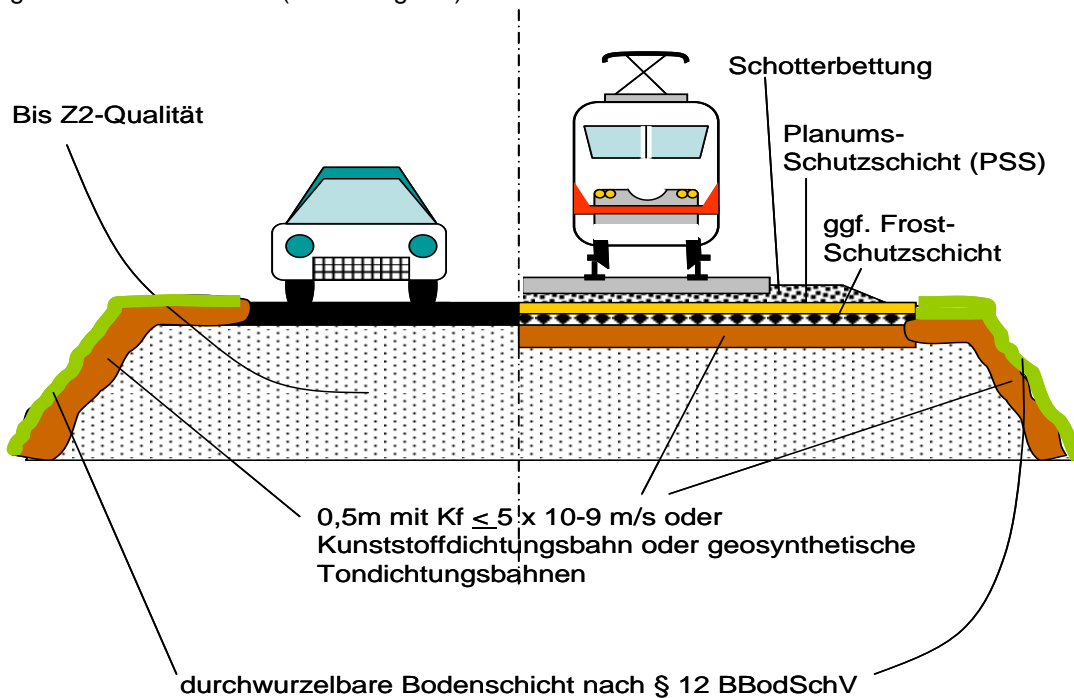
Abbildung 5-7 Regelbauweise Verkehrswegedamm
